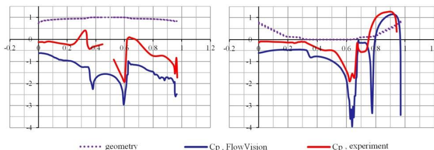
Рисунок 6. Распределение коэффициента давления C_p по поверхности профиля транспортного модуля, полученных в 2D постановке FlowVision и в эксперименте (направление набегающего потока – справа налево). Слева – по поверхности верхней части геометрии. Справа – по нижней.
