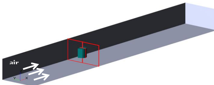
Рисунке 7. Полная трехмерная постановка задачи. Положение масштабной модели транспортного модуля внутри аэродинамической трубы (размеры трубы 1x2x14 м).
