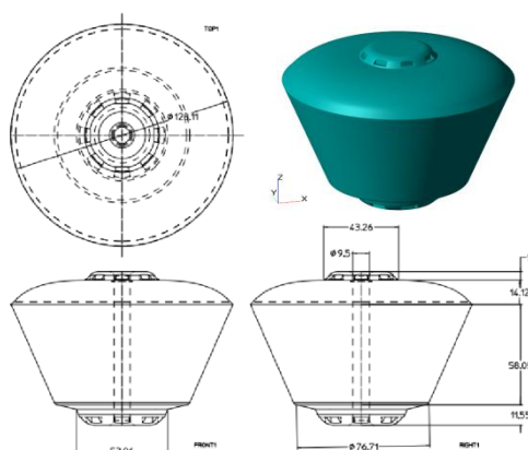
Рисунок 2. Геометрия транспортного модуля.
