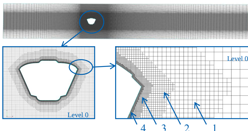
Рисунок 5. Расчетная сетка. Последовательная поверхностная адаптация: 1 уровень – 20 слоев ячеек; 2 ур. – 15; 3 ур. – 10 ; 4 ур. – 5.
