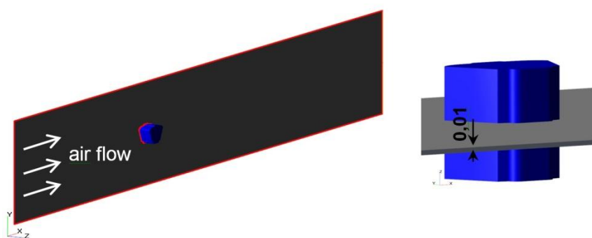
Рисунок 4. Геометрия расчетной области во FlowVision.
