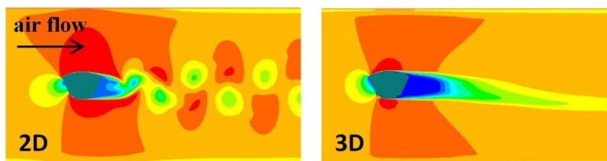
Рисунок 8. Сравнение распределения скорости [м/с] вокруг модели транспортного модуля в случае двумерной постановки задачи во FlowVision (слева) и трехмерной (справа).
