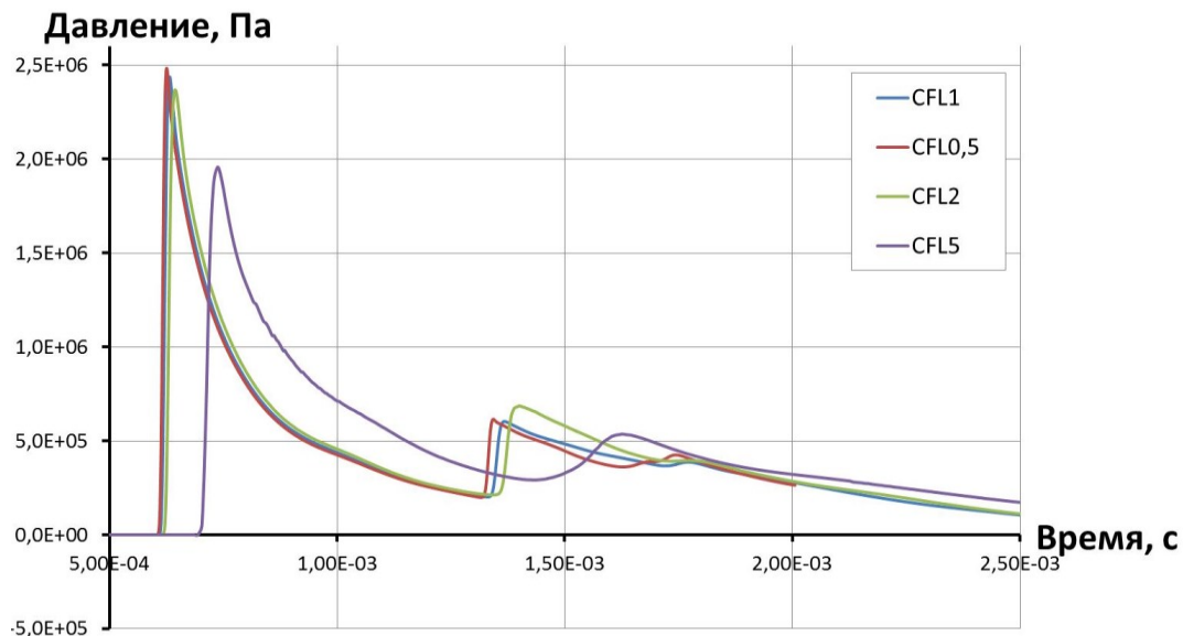
Рис.8 – Влияние шага по времени
