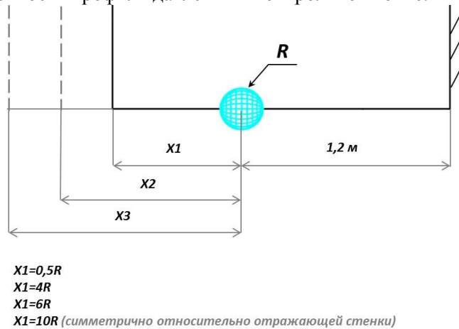
Рис.5 – Исследование конфигурации расчетной области
