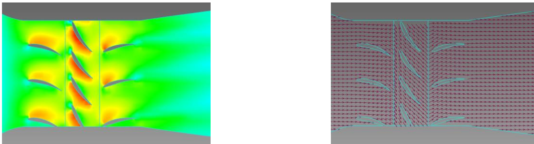
Рис. 2 – Картина течения в лопастной системе.
