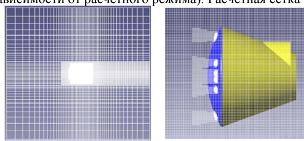
Общий вид сетки Сетка вокруг ВА Рисунок 4. Расчетная сетка для режима торможения
