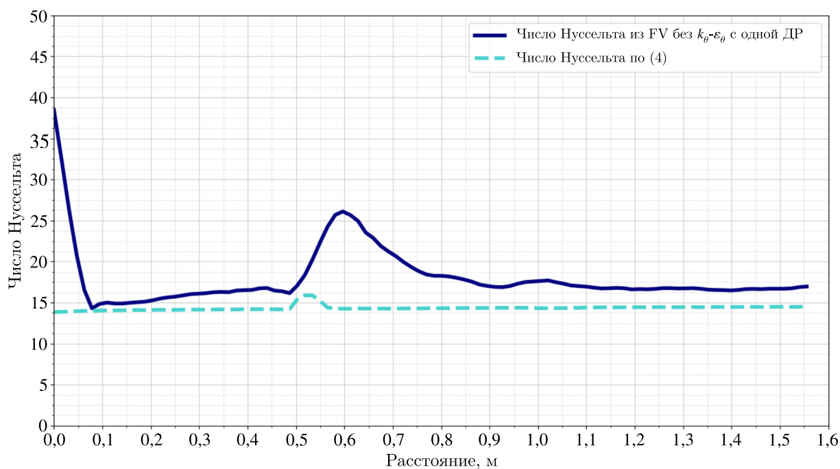
Рис. 7. Зависимость числа Нуссельта от расстояния от входа в пучок
