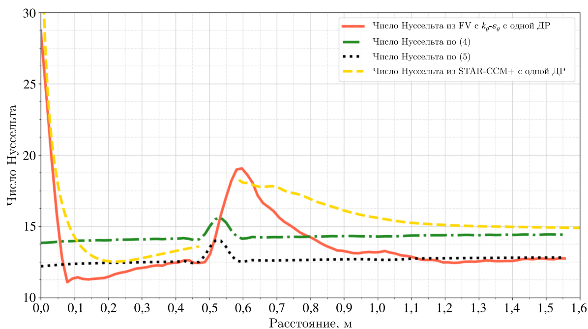
Рис. 10. Сравнение значений по корреляциям (4) и (5) с данными из FlowVision и STAR-CCM+
