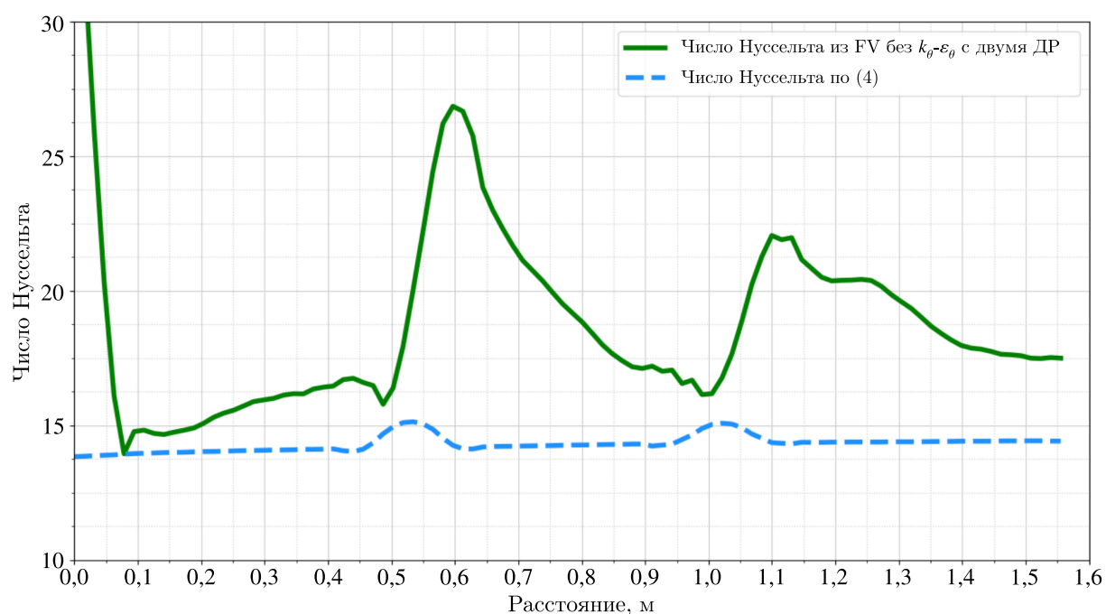
Рис. 8. Зависимость числа Нуссельта от расстояния от входа в пучок
