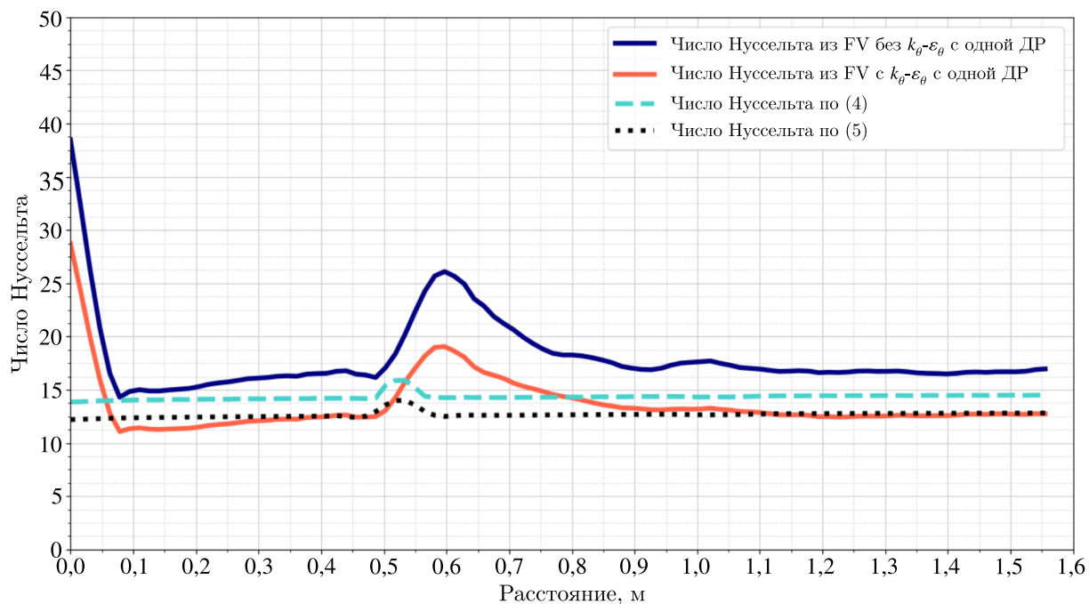
Рис. 9. Сравнение расчетов числа Нуссельта из FV с одной ДР с использованием и без k_\theta - e_\theta -модели
