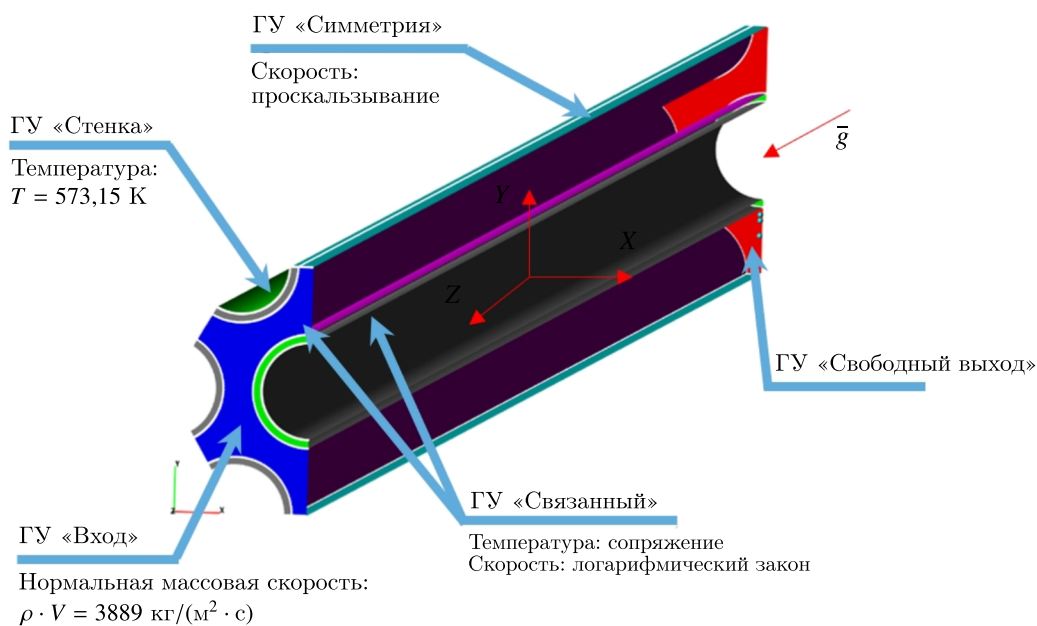
Рис. 3. Граничные условия для 3D-постановки
