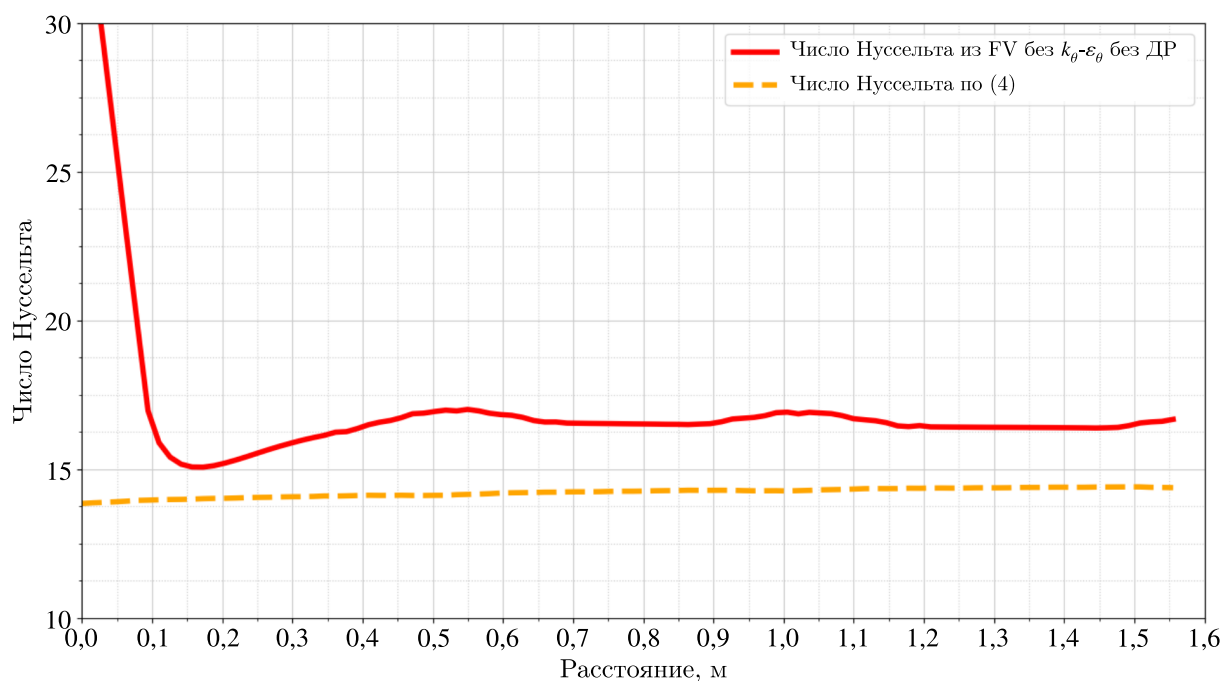
Рис. 4. График зависимости числа Нуссельта от расстояния от входа в пучок
